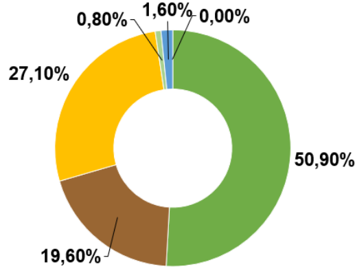
verbleibender Energieträgermix
